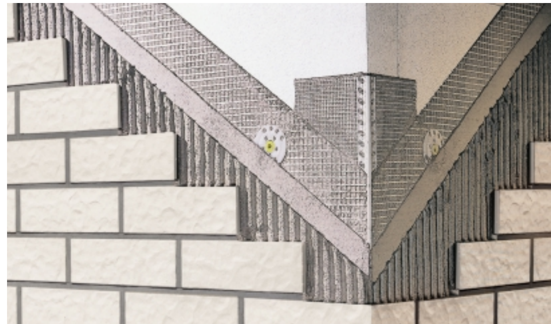
Assemblaggio di un sistema termoisolante a strati con listelli: il calore rimane all'interno dell'edificio e la facciata non avrà bisogno di manutenzione per lungo tempo.
